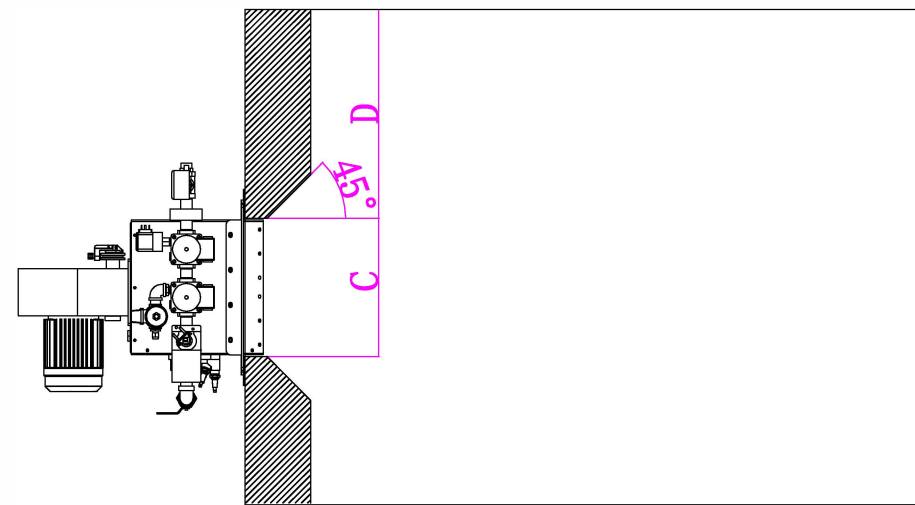
DEEVAL系列热风炉参数
